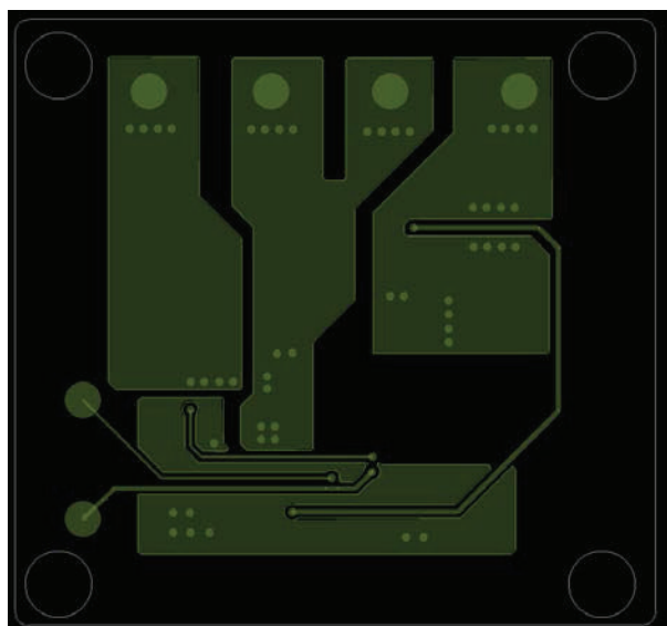
Fig. 4 - Inner Layer 2
