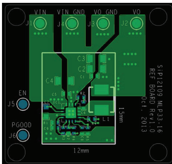
Fig. 3 - Top Layer
