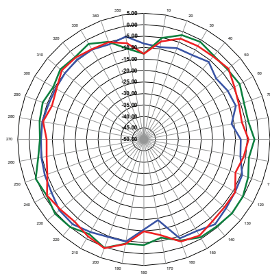
XZ-Plane Gain
