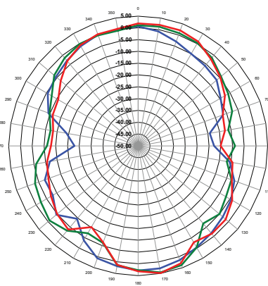
YZ-Plane Gain
