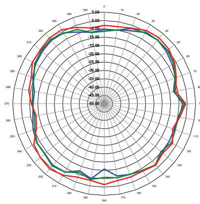
XZ-Plane Gain
