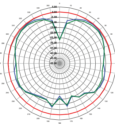
YZ-Plane Gain
