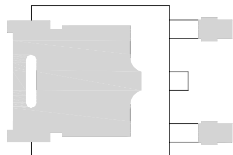
Fig. 2 - PowerPAK SO-8
