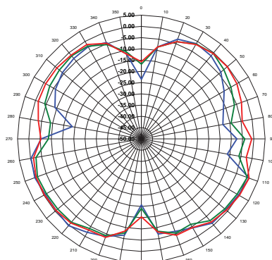
XZ-Plane Gain
