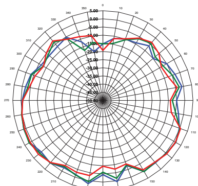
XZ-Plane Gain
