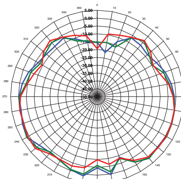
YZ-Plane Gain
