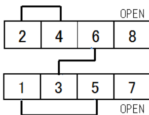
WIRING SCHEMATIC
