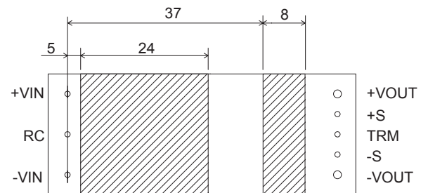
(d) CHS200
