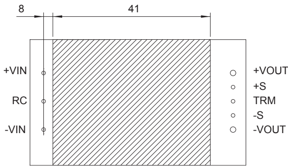
(f) CHS400/CHS500
