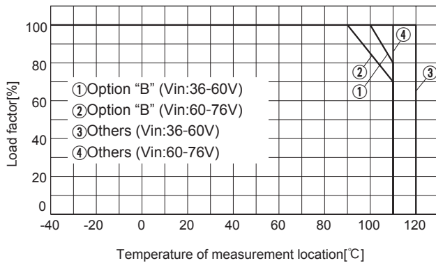
(d) CHS3804812/CHS3804812H
