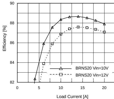
(a) Efficiency (BRNS20) BRNS20 Vo=1.2V
