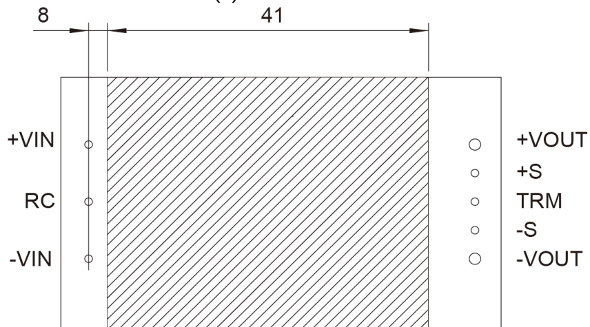
(f) CHS400 / 500
