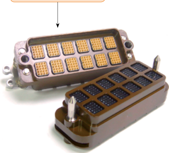
Platine métallique 12 modules 12 modules metallic plate
