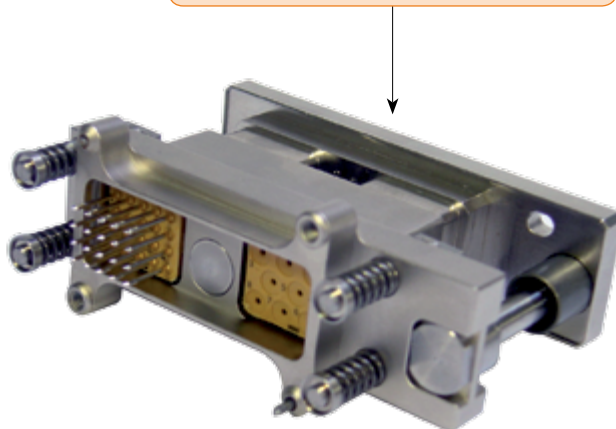
Connecteur rackable métallique 2 modules 2 modules metallic rackable connector
