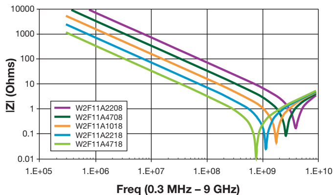
IMPEDANCE 0805 – 100V
