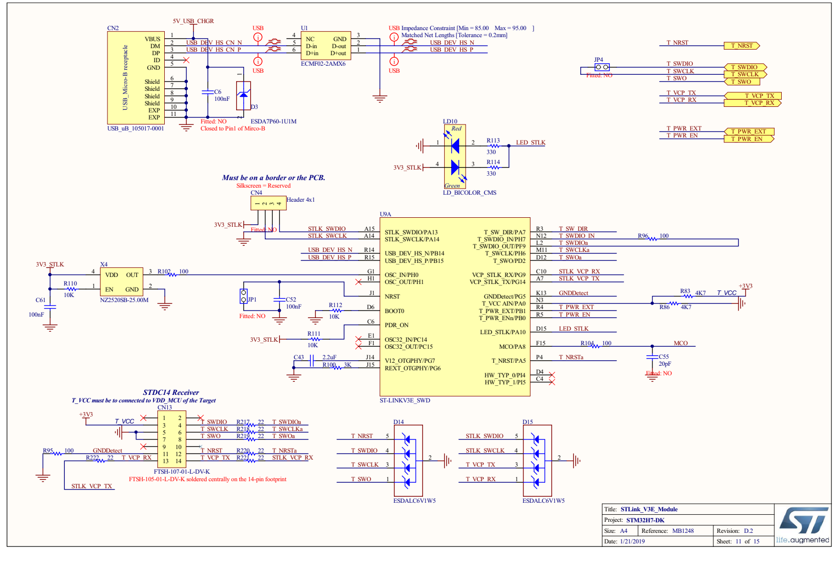
Figure 32. STLINK-V3E module
