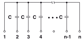
原理图 03
