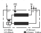
MOTOR WIRING DIAGRAMS
