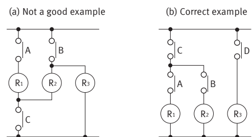
Fig. 6 Stray circuits
