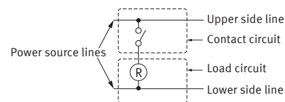
Fig. 6 Stray circuits
