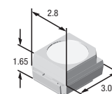
PLCC-2
