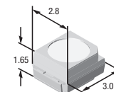
PLCC-2
