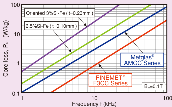
図2 各種カットコアのコアロス特性 Fig. 2 Core loss of various cut cores
