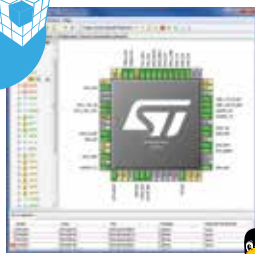
STM32CubeMX
