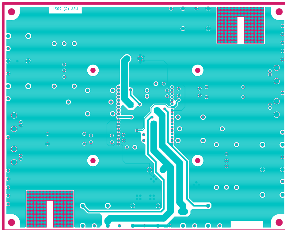
Bottom Metal Layer
