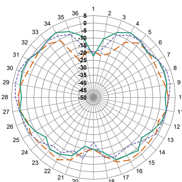
YZ-Plane Gain
