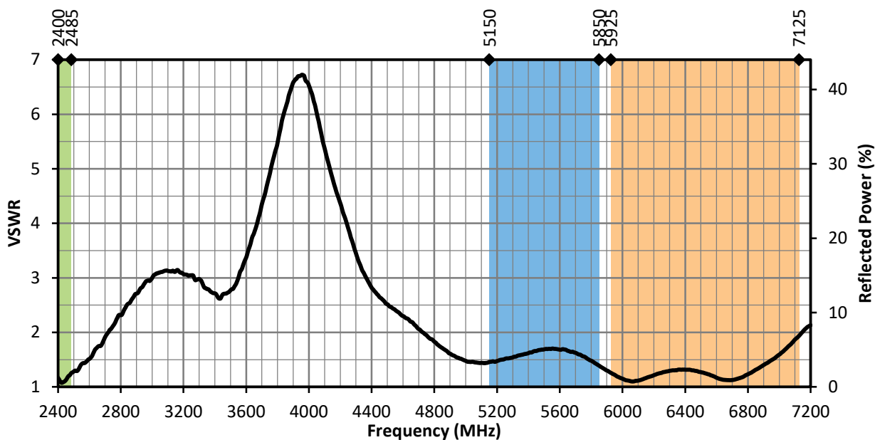
Figure 11. ANT-W63WS4-ccc VSWR, Edge-Bent
