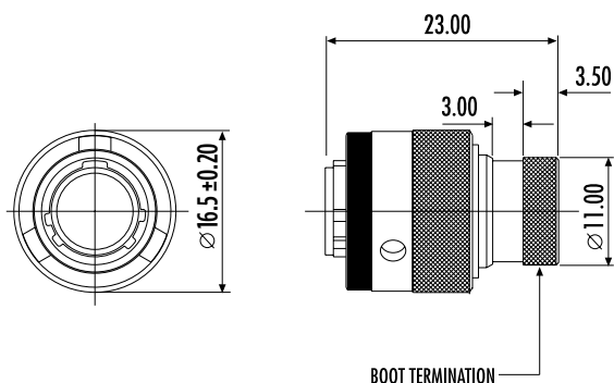
RECEPTACLE - TYPE 0
