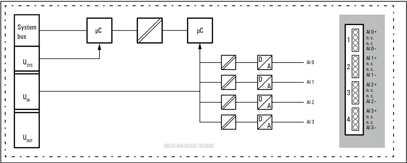
Block diagram UR20-4AI-UI-ISO-16-DIAG
