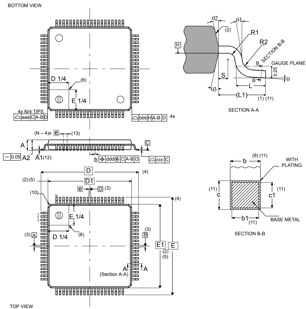
Figure 45. LQFP80 - Outline (15.)
