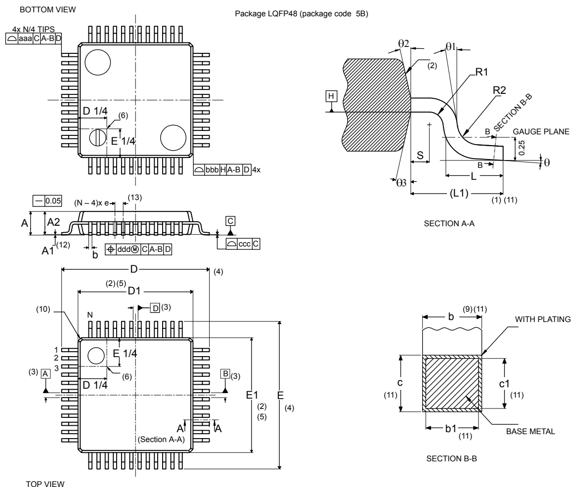
Figure 40. LQFP48- Outline (15.)
