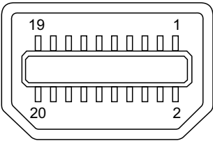
Figure 3-15: Mini DisplayPort Pin Definition
