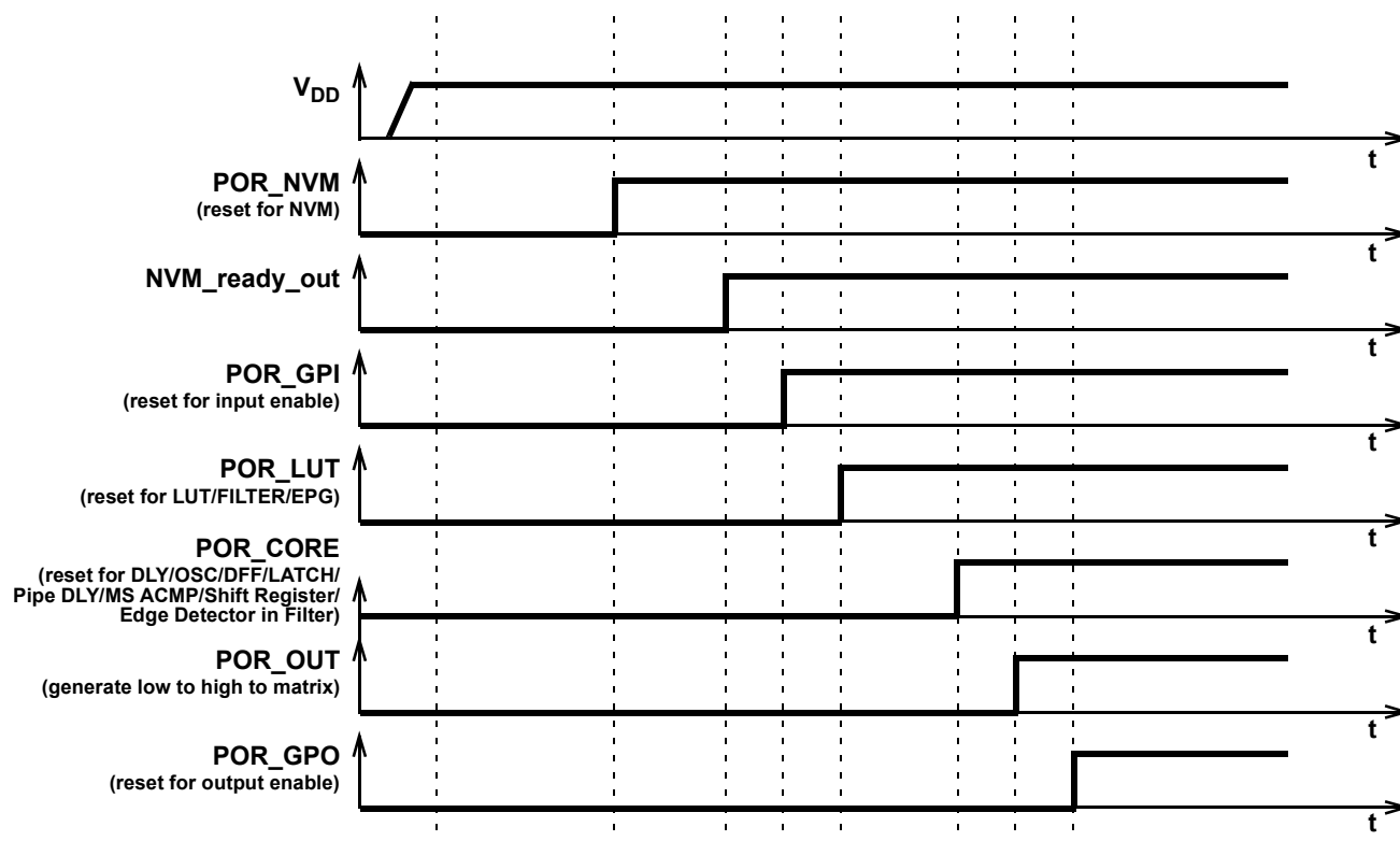
Figure 78: POR Sequence
