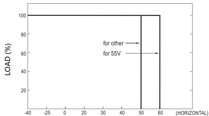
Tcase (°C)
