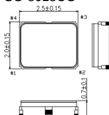
SG-8018CG
