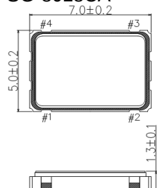
SG-8018CA
