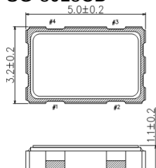
SG-8018CB
