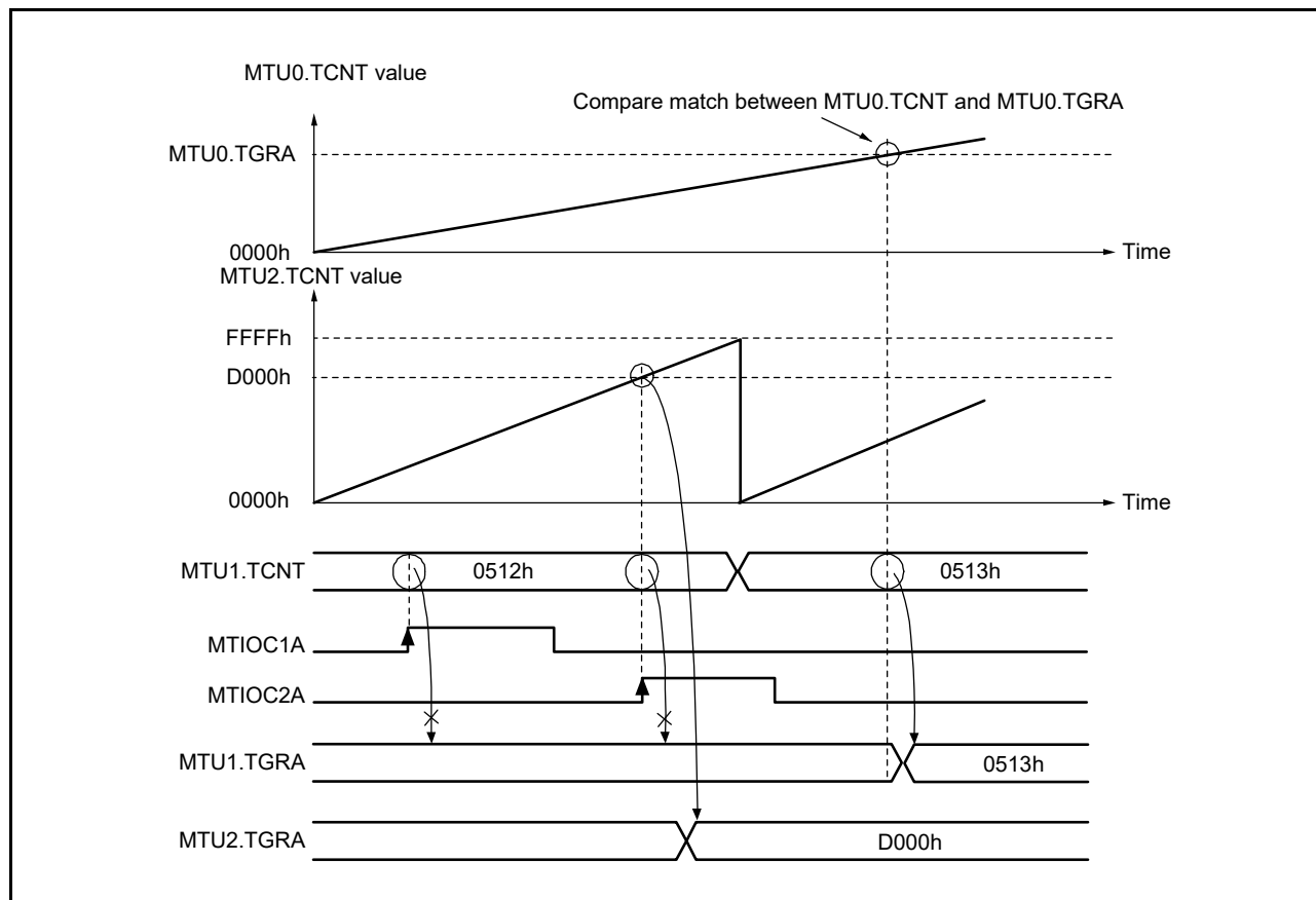
Figure 19.24 Cascaded Operation Example (d)
