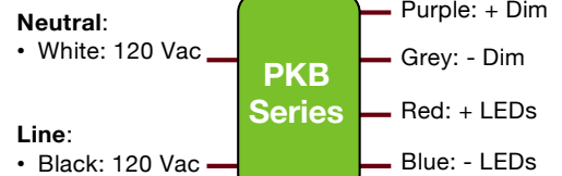
Wiring Diagrams
