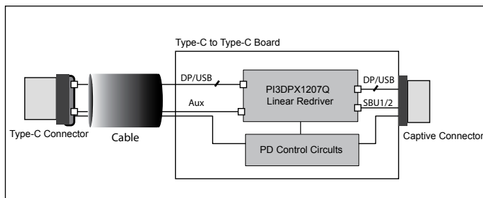
DP-AIt to DP Active Cables
