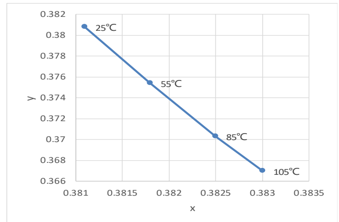
SOLDERING TEMP. VS. CIE X, Y SHIFT
