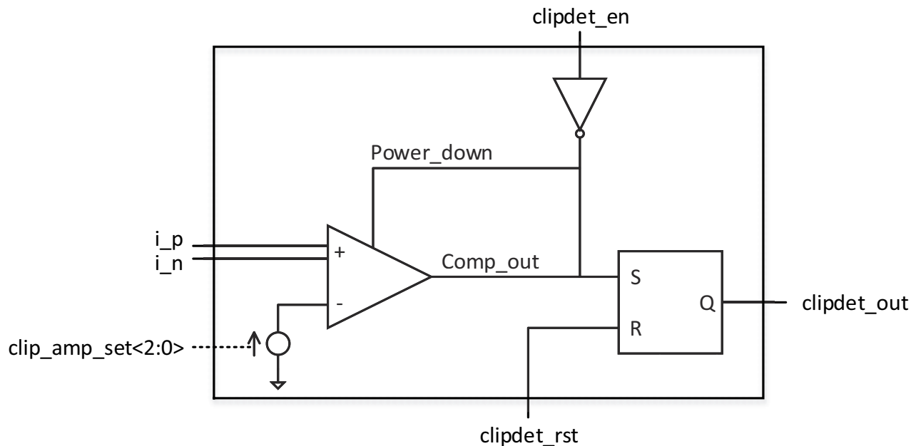
Fig 119. Clip detector 1
