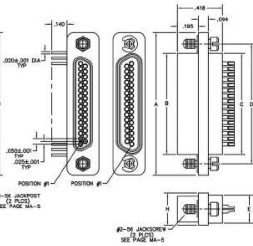
RECEPTACLE
