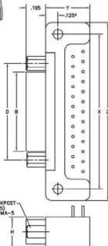
RECEPTACLE
