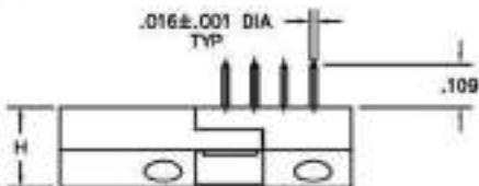
RECEPTACLE
