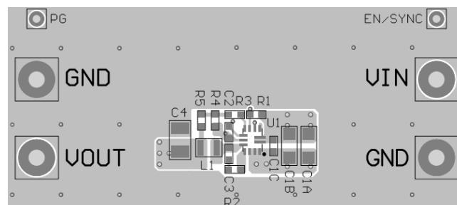
Top Layer
