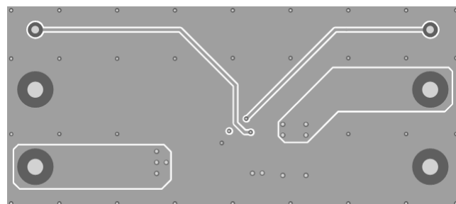
Inner Layer 2
