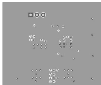
Bottom Layer
