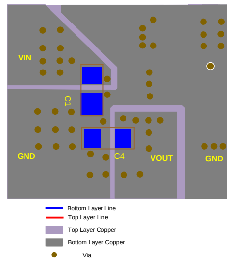
Bottom Layer
