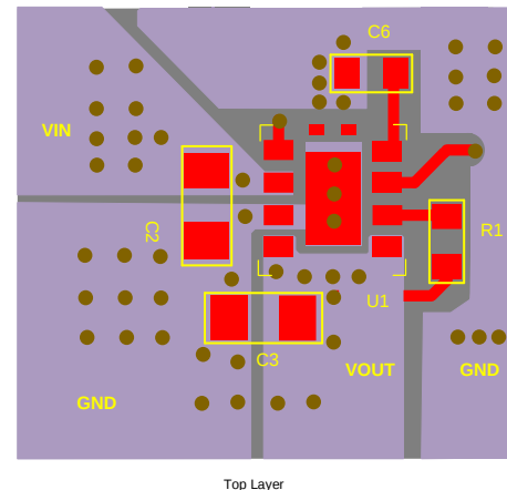
Top Layer
