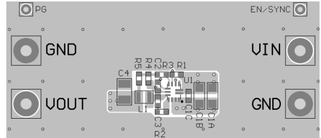
Top Layer
