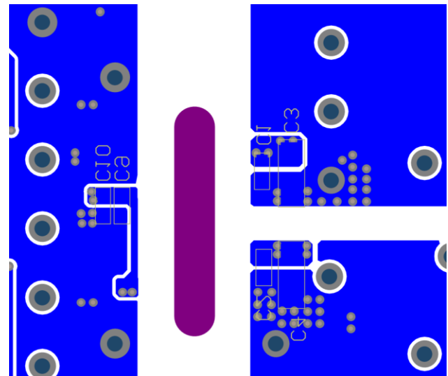
Top Layer
