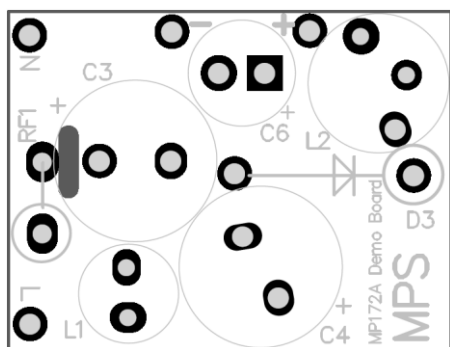
Top Layer
