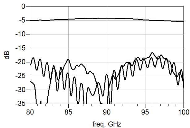
Thru S-Parameters
