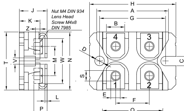
L027a SOT-227 B miniBLOC
