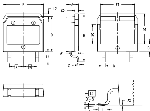
L019a TO-268 AA (D*PAK HV)
