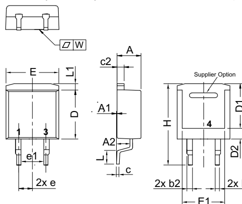
X011c TO-263 AB (D 2 PAK HV)
