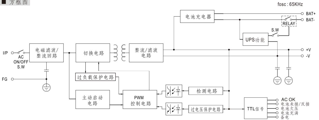
■ 方框图
