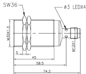
Fig. 20 Flush version, plug
