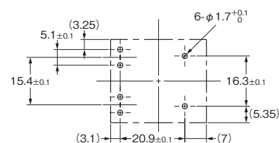
取り付け穴加工寸法
