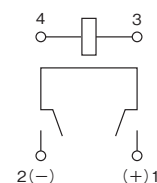
端子配置／内部接続図
