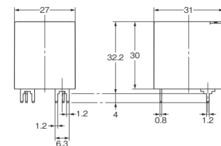
基板取り付け状態(参考)
