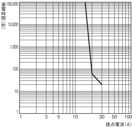
●通電電流－通電時間曲線
