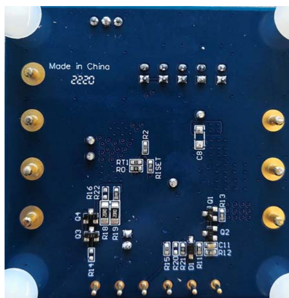
Bottom Layer
