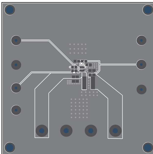
Figure 4—Top Layer
