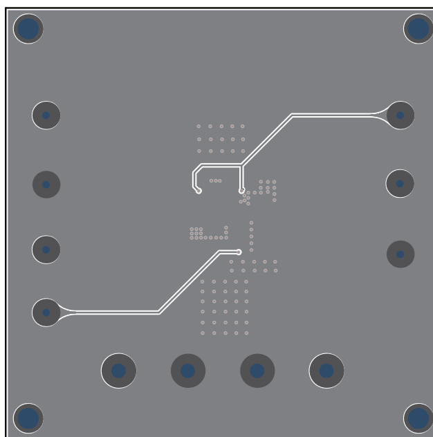
Figure 5—Bottom Layer
