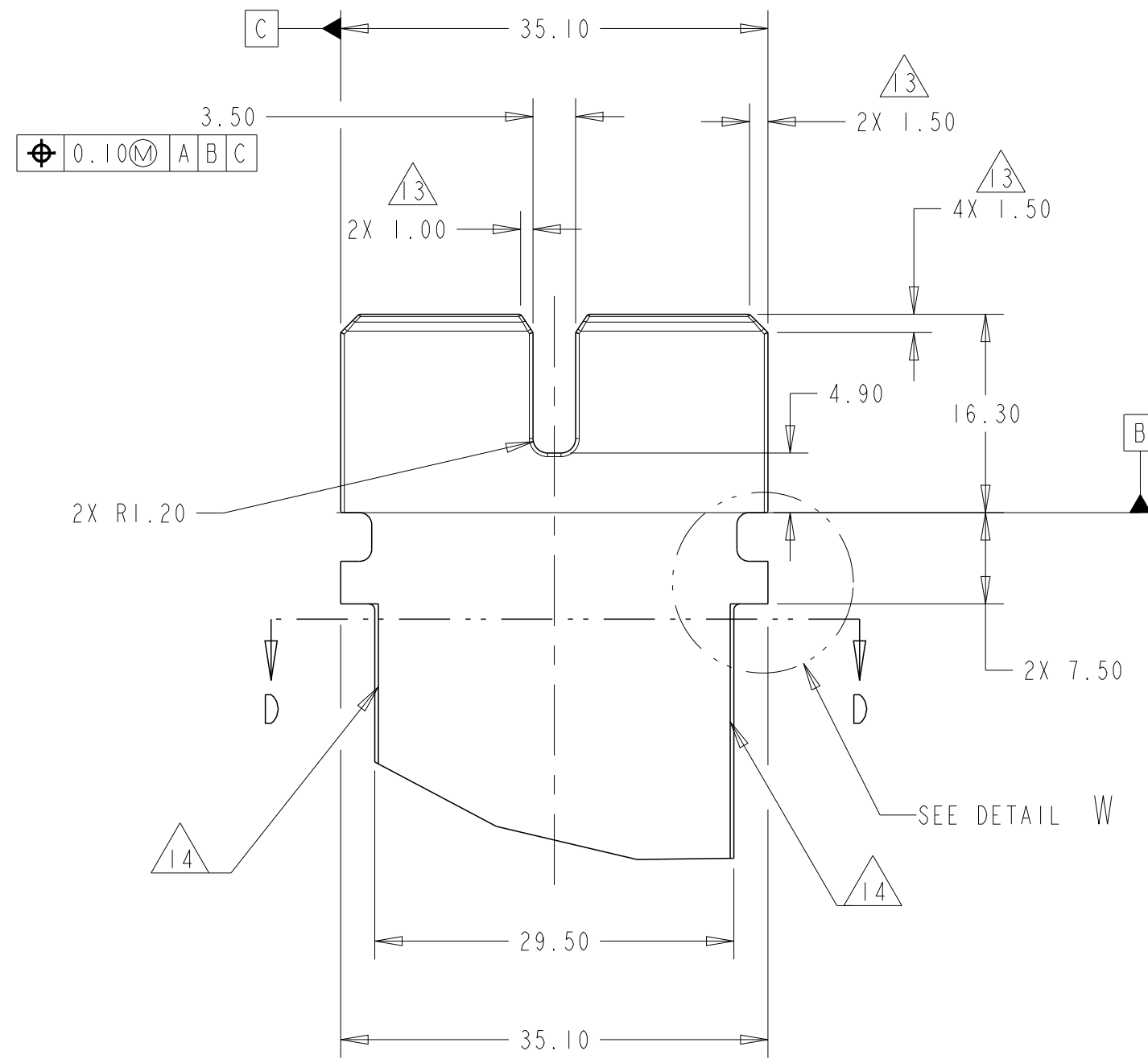
HEADER TAB INTERFACE SCALE 2:1
