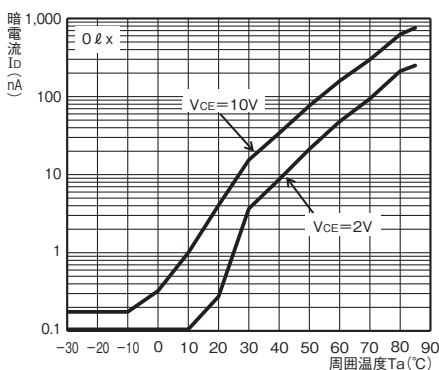
図6. 暗電流—周囲温度特性 (TYP.)
