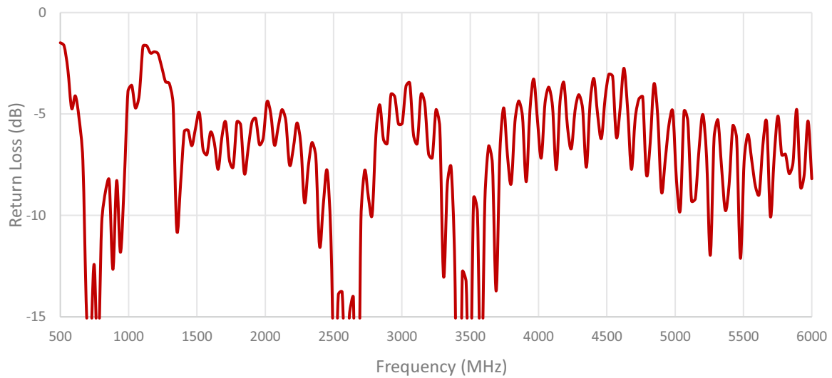
Cable 1: 5GNR
