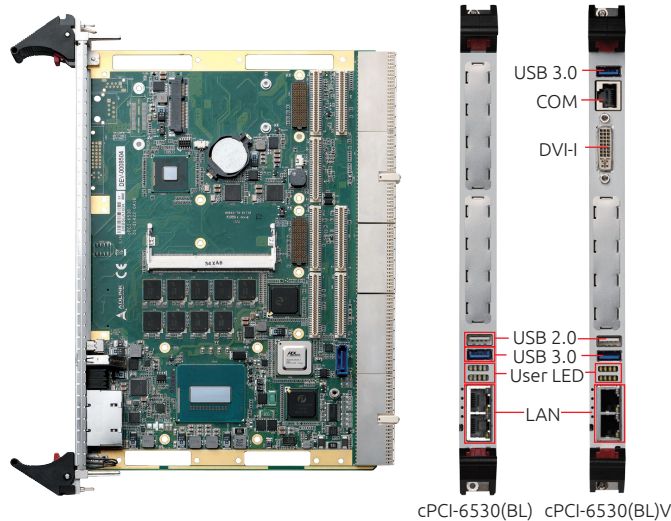
cPCI-6530(BL) cPCI-6530(BL)V
