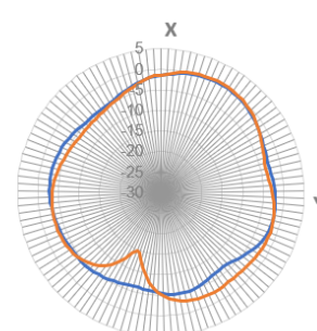
— 1575 MHz — 1602 MHz
