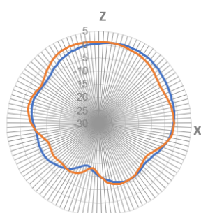
— 1575 MHz — 1602 MHz
