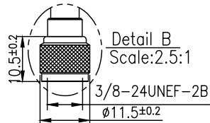
Mini UHF(M)ST Plug
